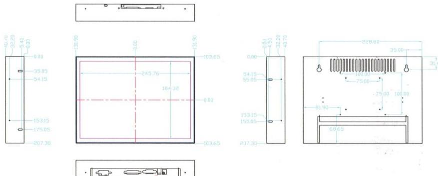
12.1六视尺寸图
